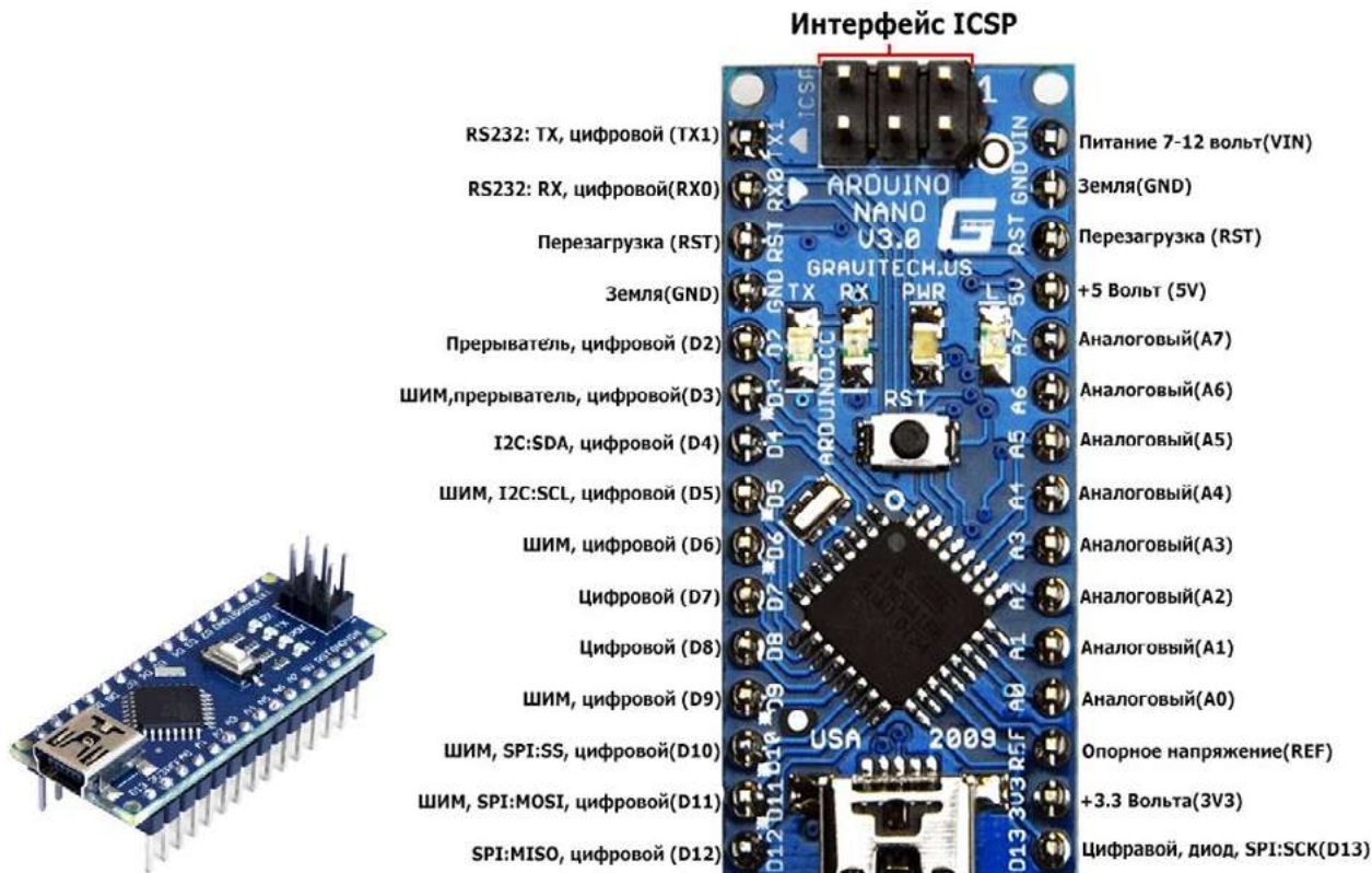
Рис. 120. Плата Arduino-нано
